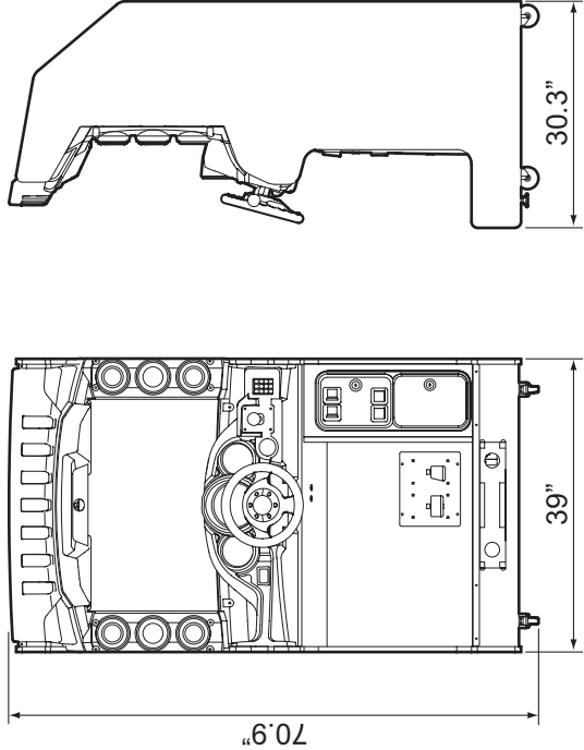
Front assembly Width (W) 39" × depth (D) 30.3" × height (H) 70.9"
